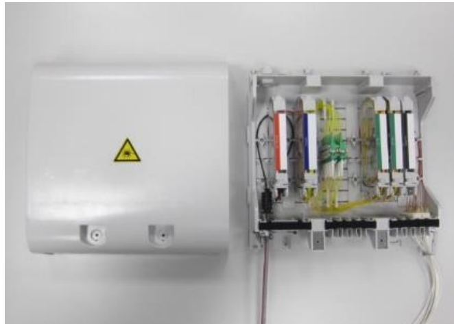
HÜP - Gebäudeanschluss Hausanschluss-Raum Beispiel einer One Box (Glasfaser Abschlusspunkt)
